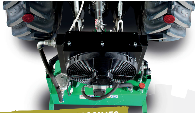
SUPPORTO MOTORI SAGOMATO IN TECNOPOLIMERO AD ALTA RESISTENZA
